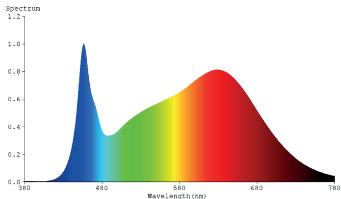
Spektrální graf MZ-CCT-1920-24V (2200 K + 6500 K)
